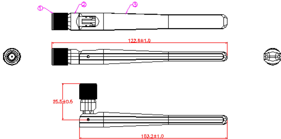
<Bar Type 외장 안테나>
